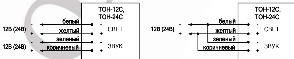
Рис.1. Схема подключения.
